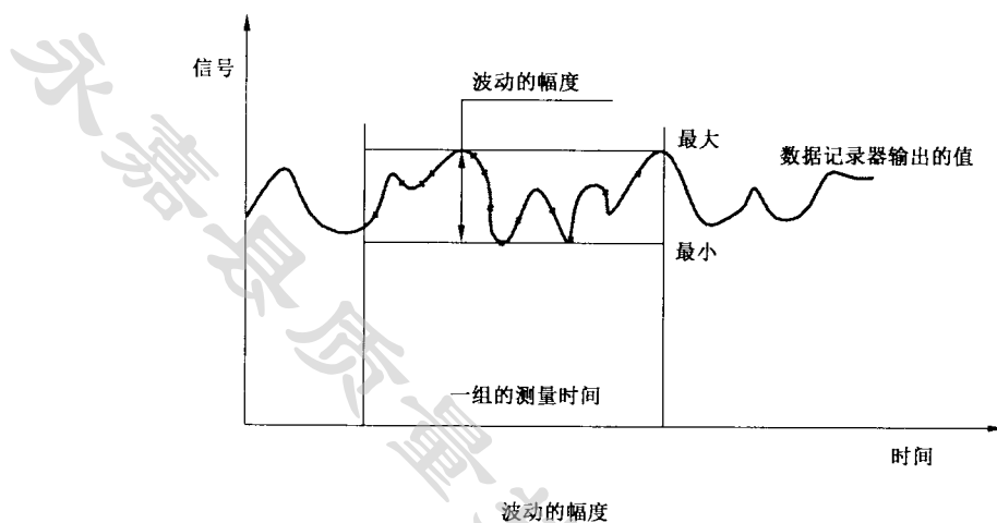
图 B.2 波动的幅度
