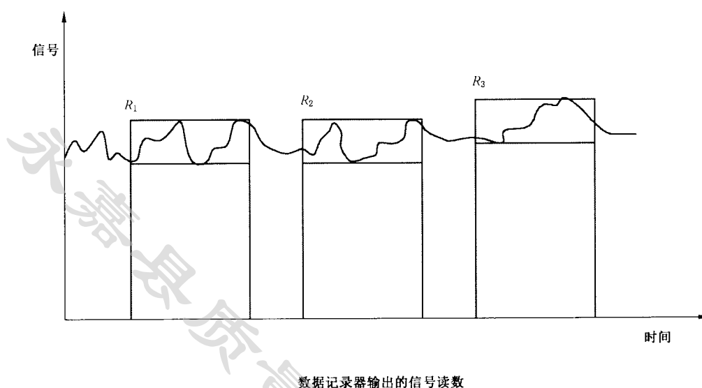
图 B.3 数据记录器输出的信号读数
